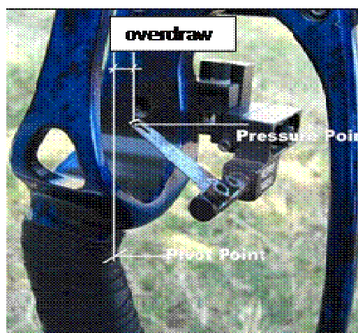
Un exemple de repose flèche (arc système) avec un dispositif d'overdraw
